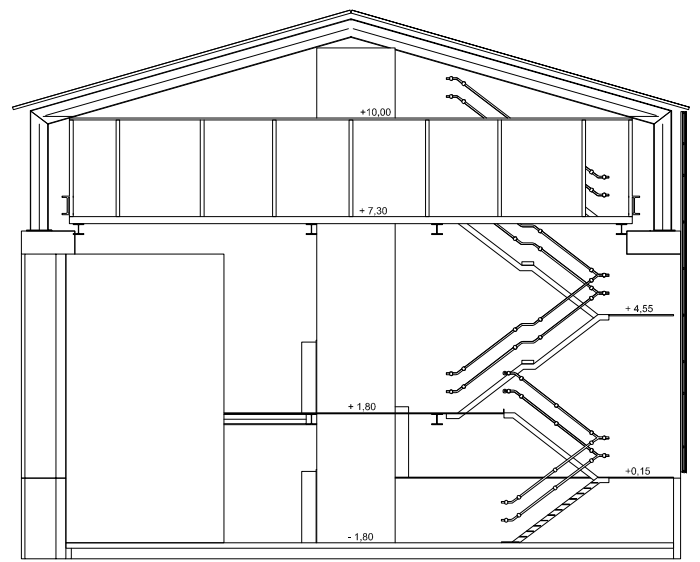
B-B
